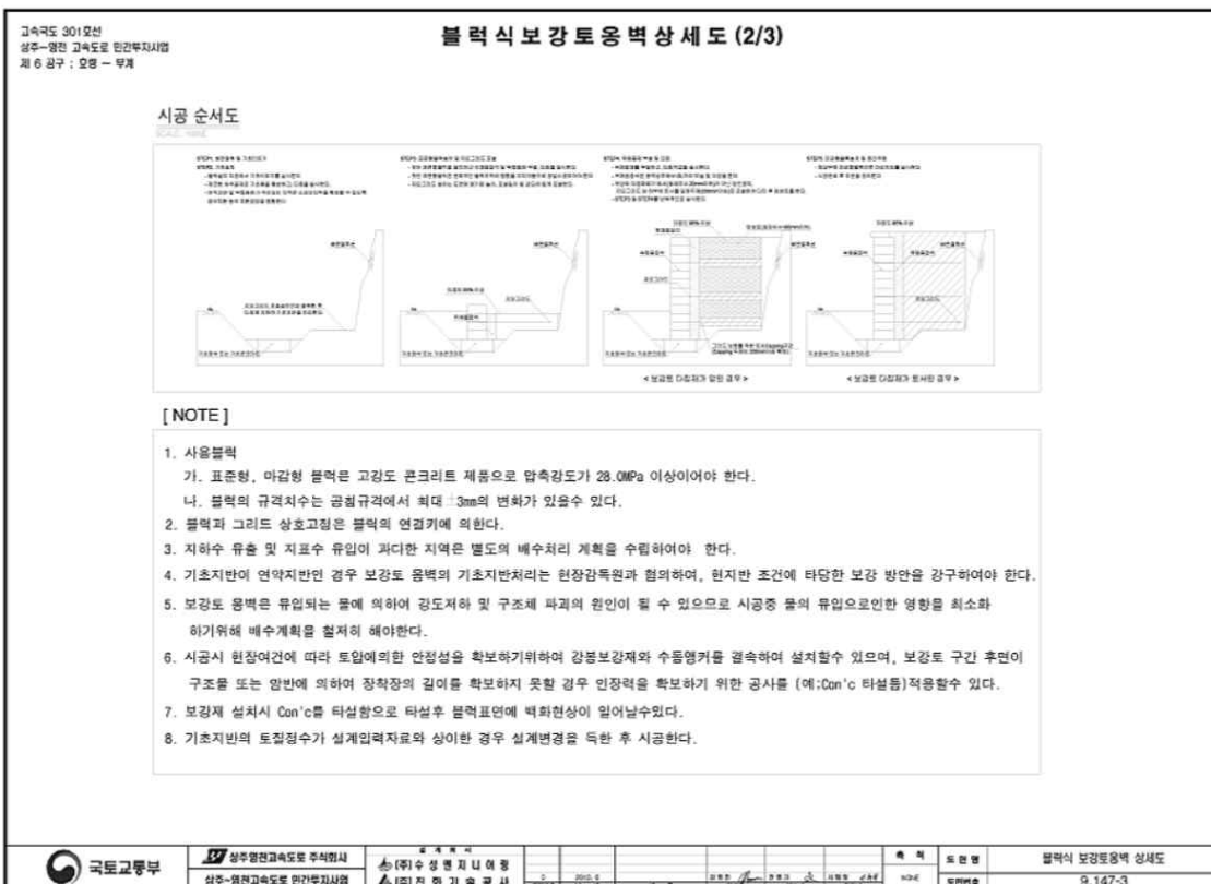
【그림 70.6】 상세도
