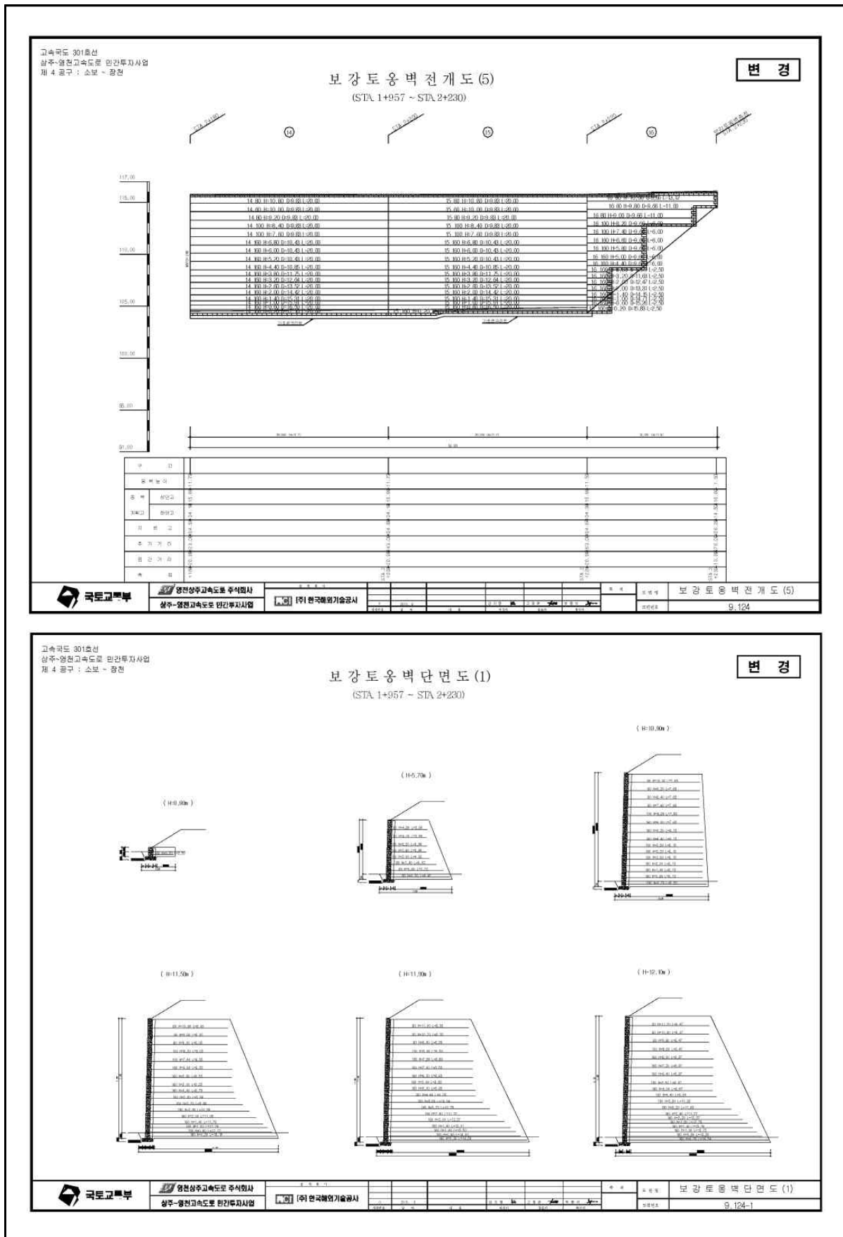
【그림 70.5】전개도 및 단면도
