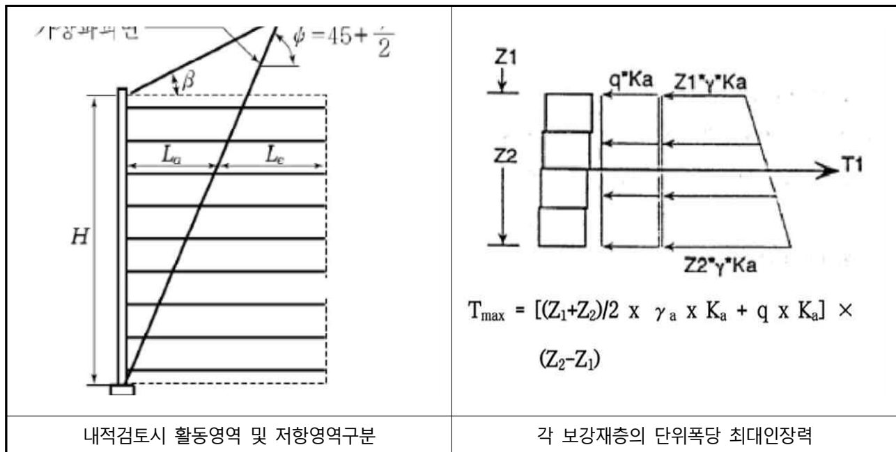
【그림 70.13】 토압작용 모식도
