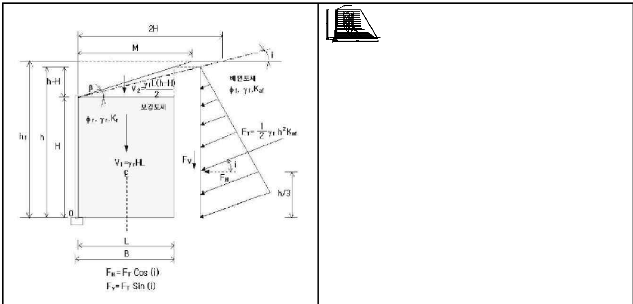
【그림 70.12】 검토단면도
